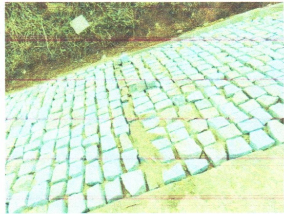
FOTO 3: TRECHO CONCLUÍDO - LADEIRA ZÉ BUCHUDO – RE CRAVA A CADA 30M;
